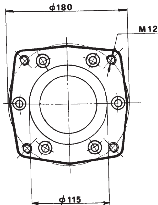
Linde Guldner PF 75 30463
