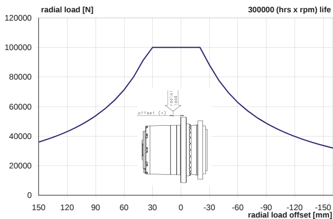
Carico radiale / Radial load
